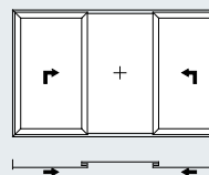
Tipo 1D.i Scorrevole internamente
